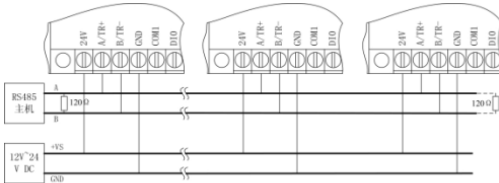
图 3.2 电源和通讯线连接
