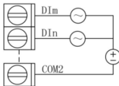
图 3.4 开关信号输出
