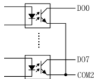
图 2.2 开关量输出电路
