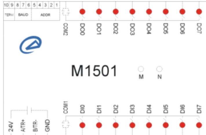
图 3.5 M1501 端子与拨码开关排列
