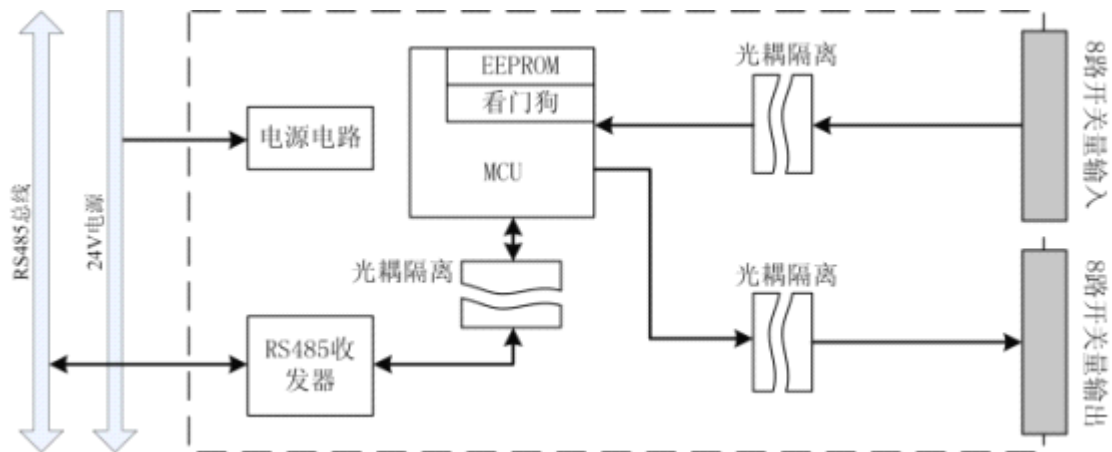
图 1.1 M1501 原理框图
