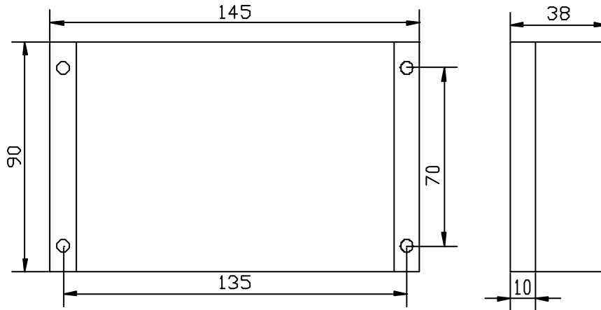
图 1.3 模块尺寸
