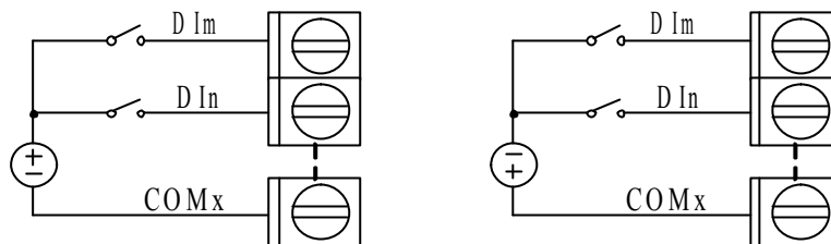
图 3.3 开关信号输入
