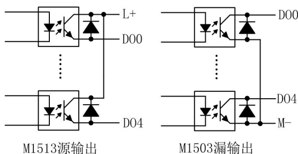
图 2.3 开关量输出电路
