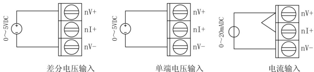
图 3.2 模拟信号输入
