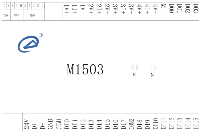
图 3.6 M1503 端子与拨码开关排列
