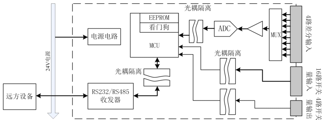
图 1.1 M1513-R 原理框图
