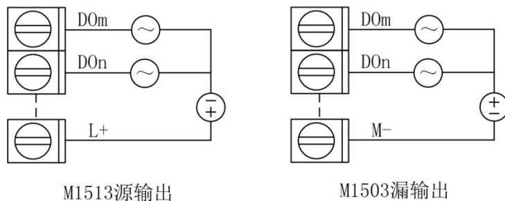
图 3.4 开关信号输出
