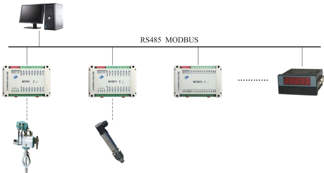
图 6.1 M1508 应用示例
