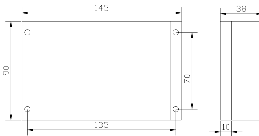
图 1.3 模块尺寸
