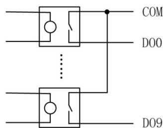
图 2.2 开关量输出电路
