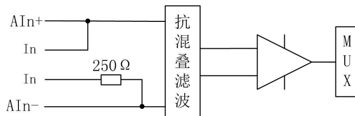
图 2.1 模拟量输入电路
