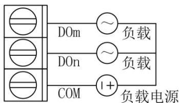
图 3.4 开关信号输出
