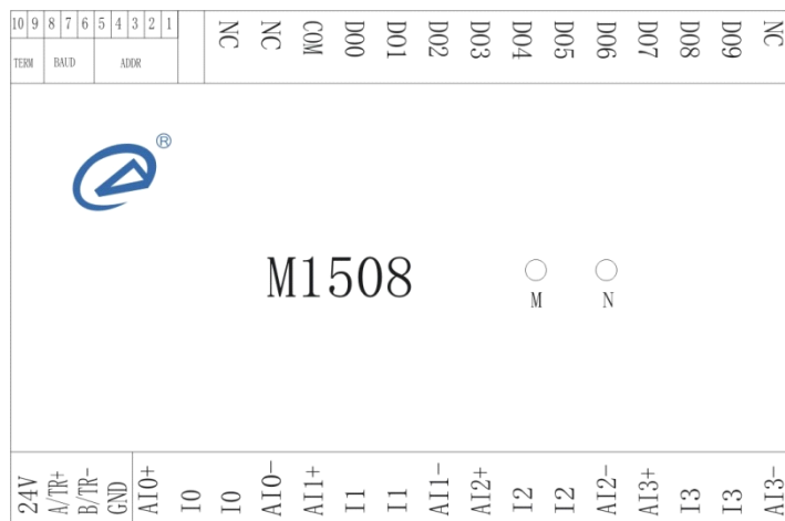
图 3.5 M1508 端子与拨码开关排列
