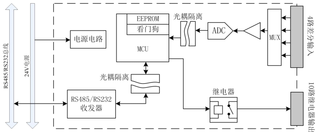
图 1.1 M1508 原理框图
