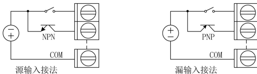
图 3.3 开关信号输入
