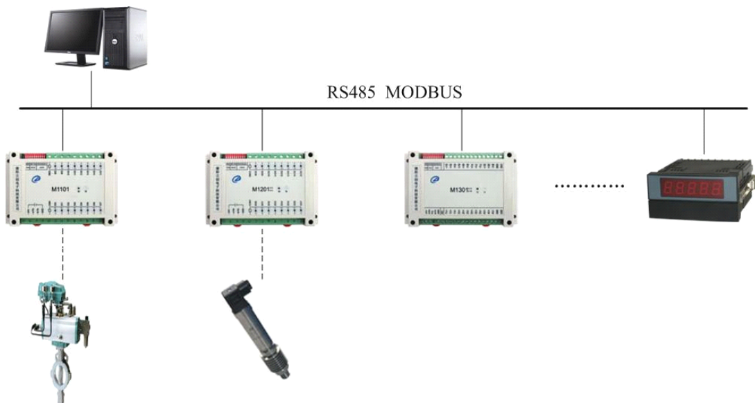
图 6.1 M1501 应用示例
