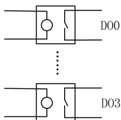
图 2.2 开关量输出电路
