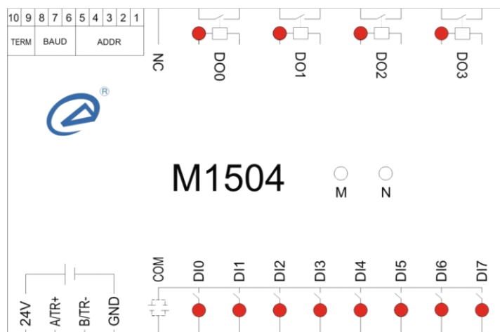
图 3.5 M1504 端子与拨码开关排列
