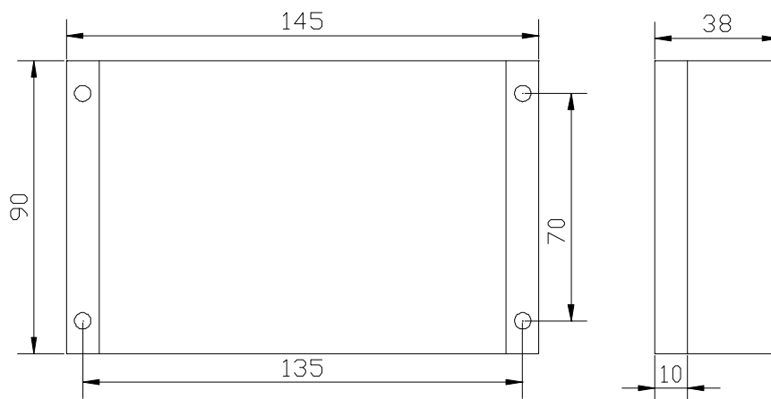
图 1.3 模块尺寸
