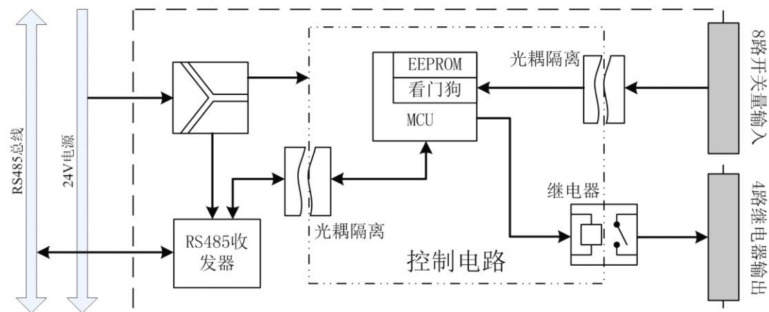
图 1.1 M1504 原理框图
