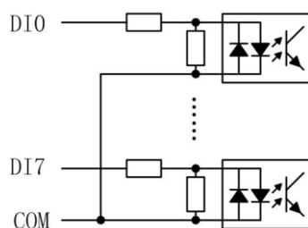
图 2.1 开关量输入电路
