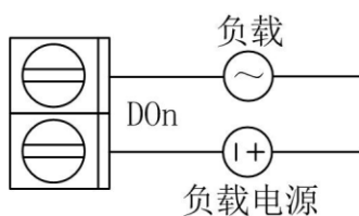
图 3.4 开关信号输出
